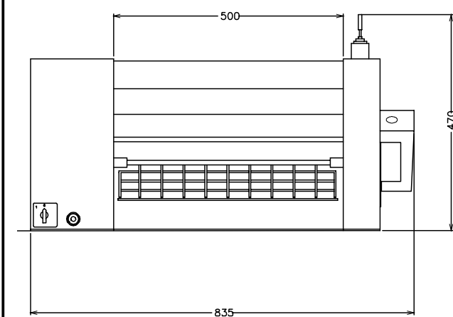
Côté
